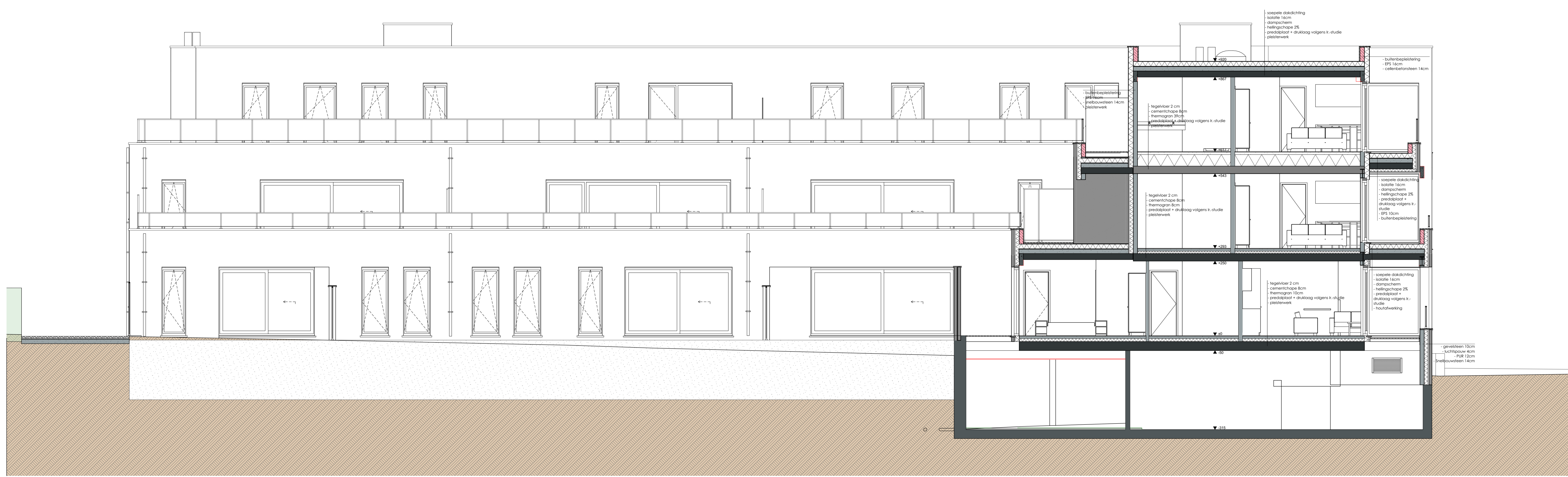
Doorsnede C-C
